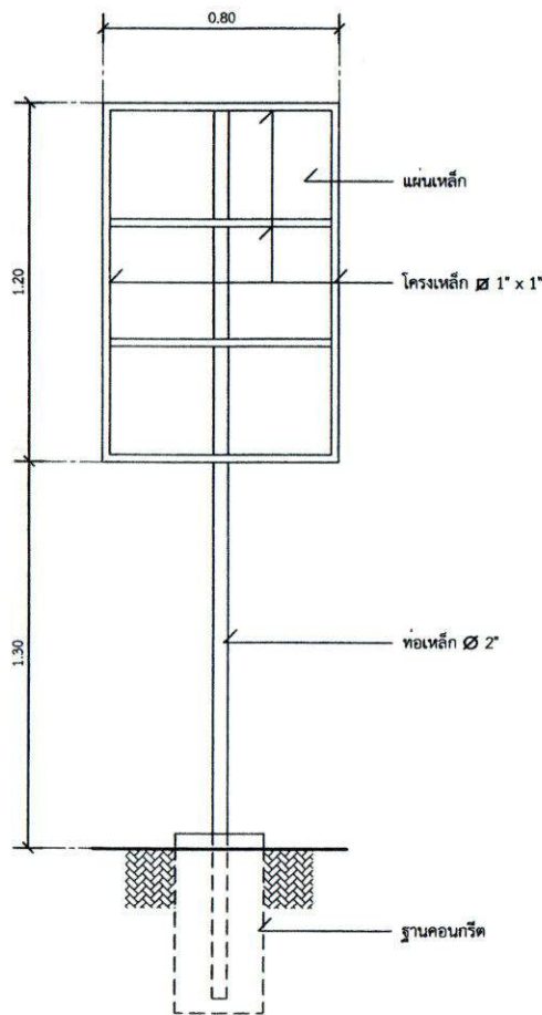
รูปด้านหลัง มาตรฐาน 1 : 20
