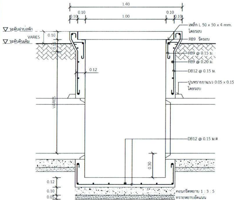
รูปตัด ก-ก 1 : 20
