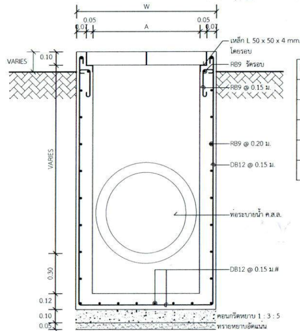
รูปตัด ข-ข 1 : 20
