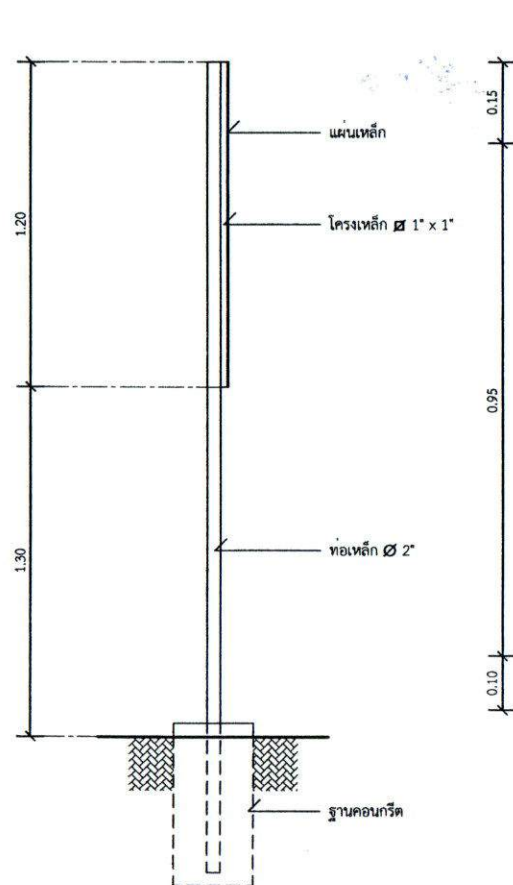
รูปด้านข้าง มาตรฐาน 1 : 20
