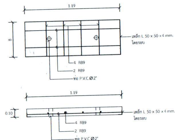
แบบขยายผ้าบ่อพัก
