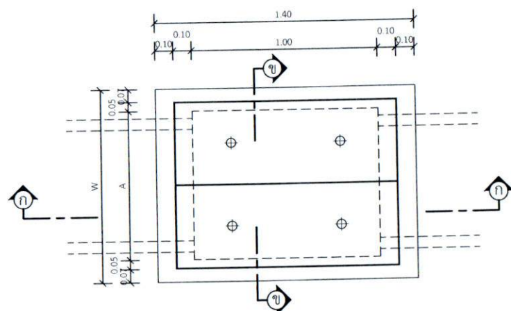
แปลนบ่อพัก ค.ส.ล.
