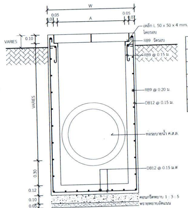
แบบขยายผ้าบ่อพัก
