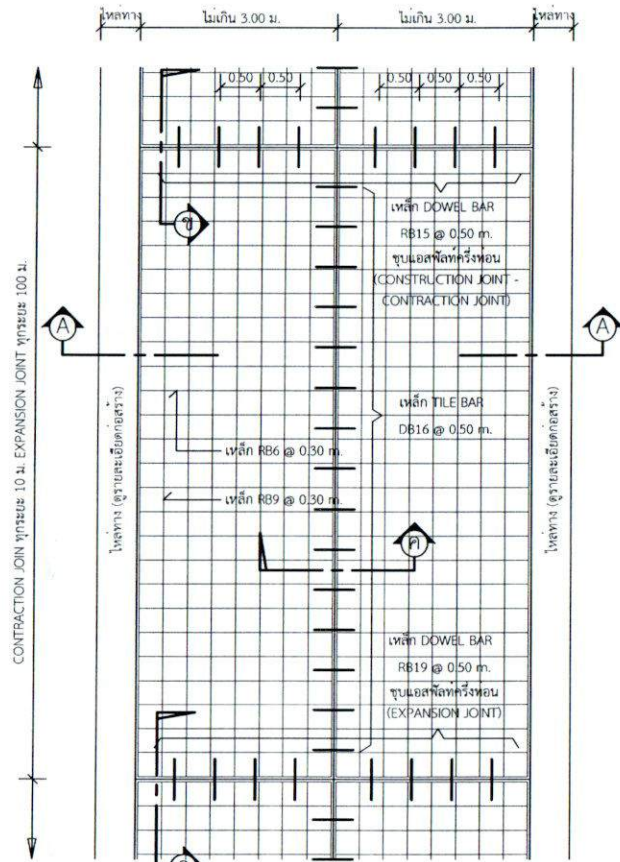
แปลนพื้นถนน
