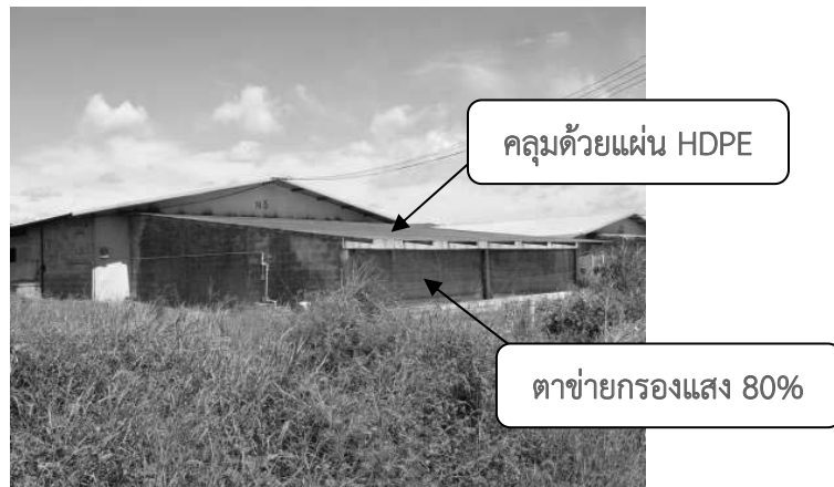
รูปที่ 7.3-18 แสดงลักษณะภายนอกของระบบกรงกลั่นมันน้ำกระจายเต็มพื้นที่
